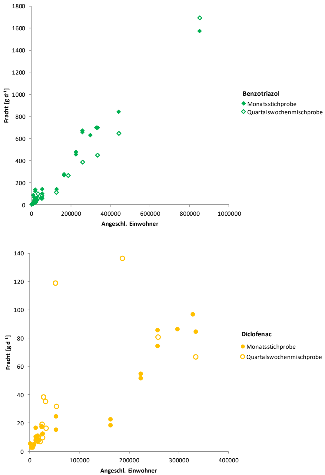
Abbildung 3.3 Mittlere tägliche Frachten von Benzotriazol (oben) und Diclofenac (unten) versus der Anzahl angeschlossener Einwohner.
