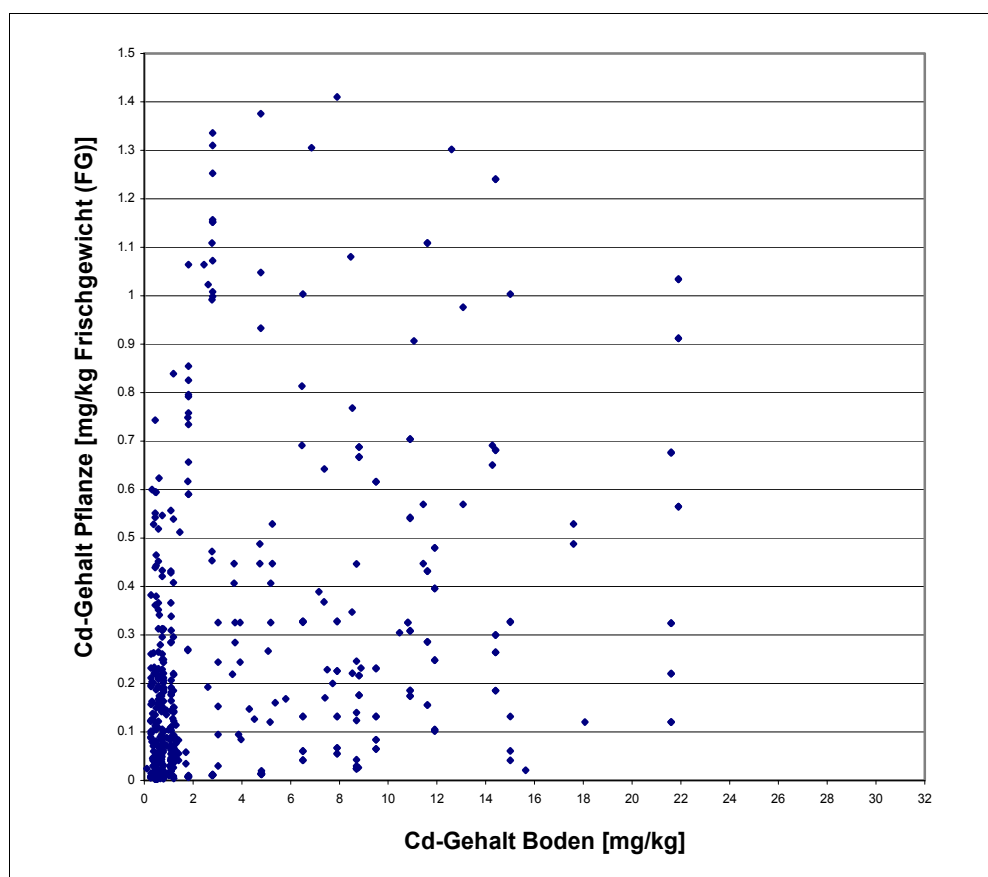
Abb. 9: Darstellung der Cd-Gehalte in Böden und Pflanzen. Faktoren: Pflanzen mit starker Cd-Aufnahme (Pflanzenartfaktor = 2, pH 5.75–6.75, Gehalt an organischer Substanz ≤8%).
