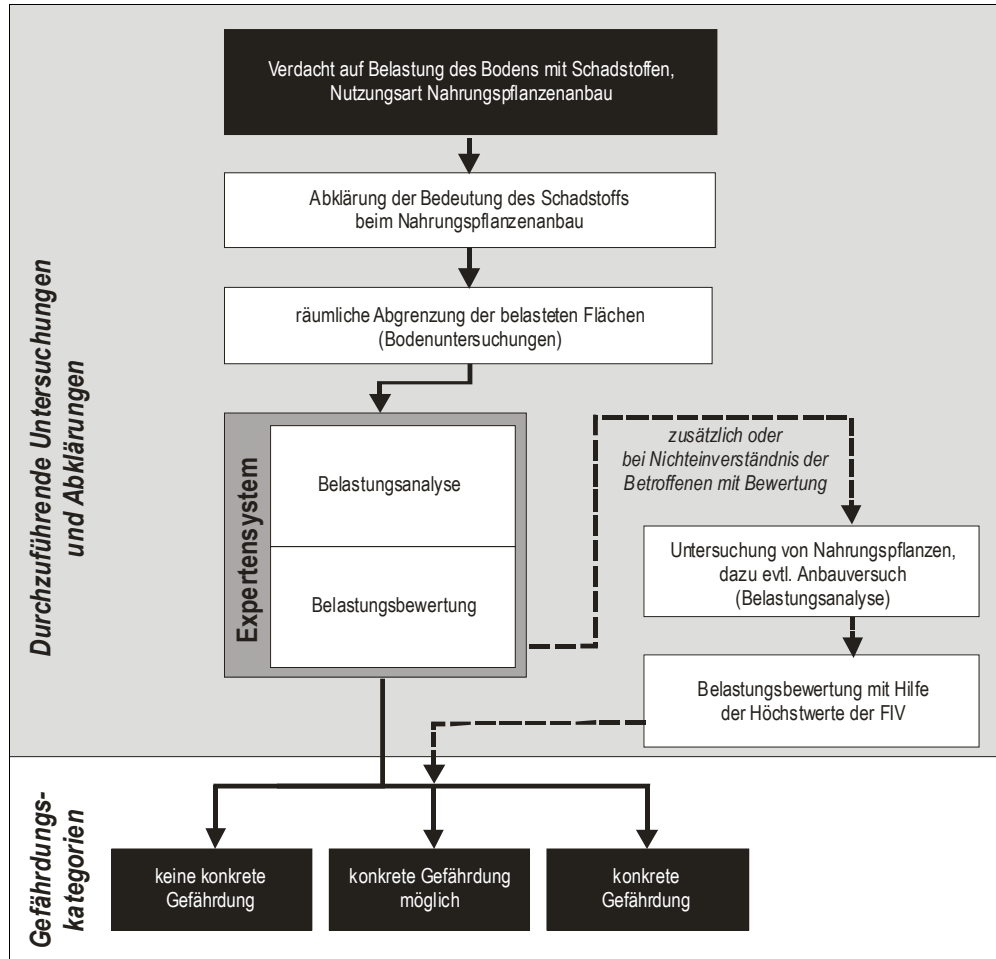
Abb. 3: Das Vorgehen in der Gefährdungsabschätzung beim Nahrungspflanzenanbau [FIV: Fremd- und Inhaltsstoffverordnung; SR 817.021.23].
