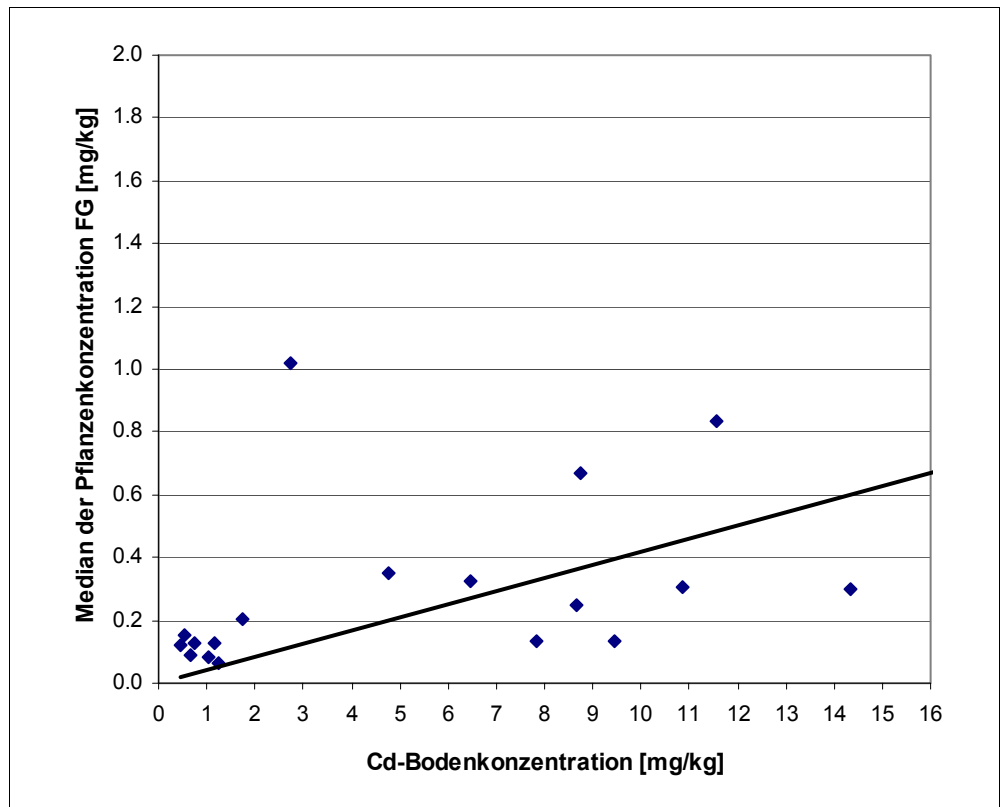
Abb. 10: Darstellung der Mediane der Cd-Gehalte in Pflanzen für Abschnitte der Bodengehalte von 0.1 mg/kg (0.0–0.1, 0.1–0.2 mg/kg) und deren lineare Korrelation. Mediane wurden nur aufgetragen, wenn für einen Abschnitt mindestens neun Messwerte vorlagen.
