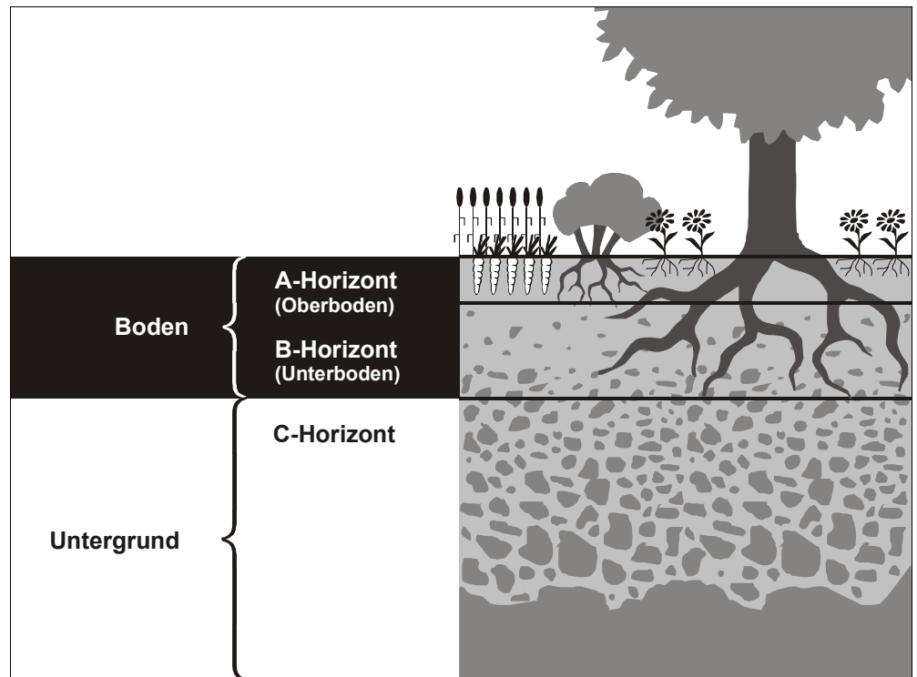
Abb. 1: Gegenstand des Handbuchs ist der mit «Boden» bezeichnete Bereich.
