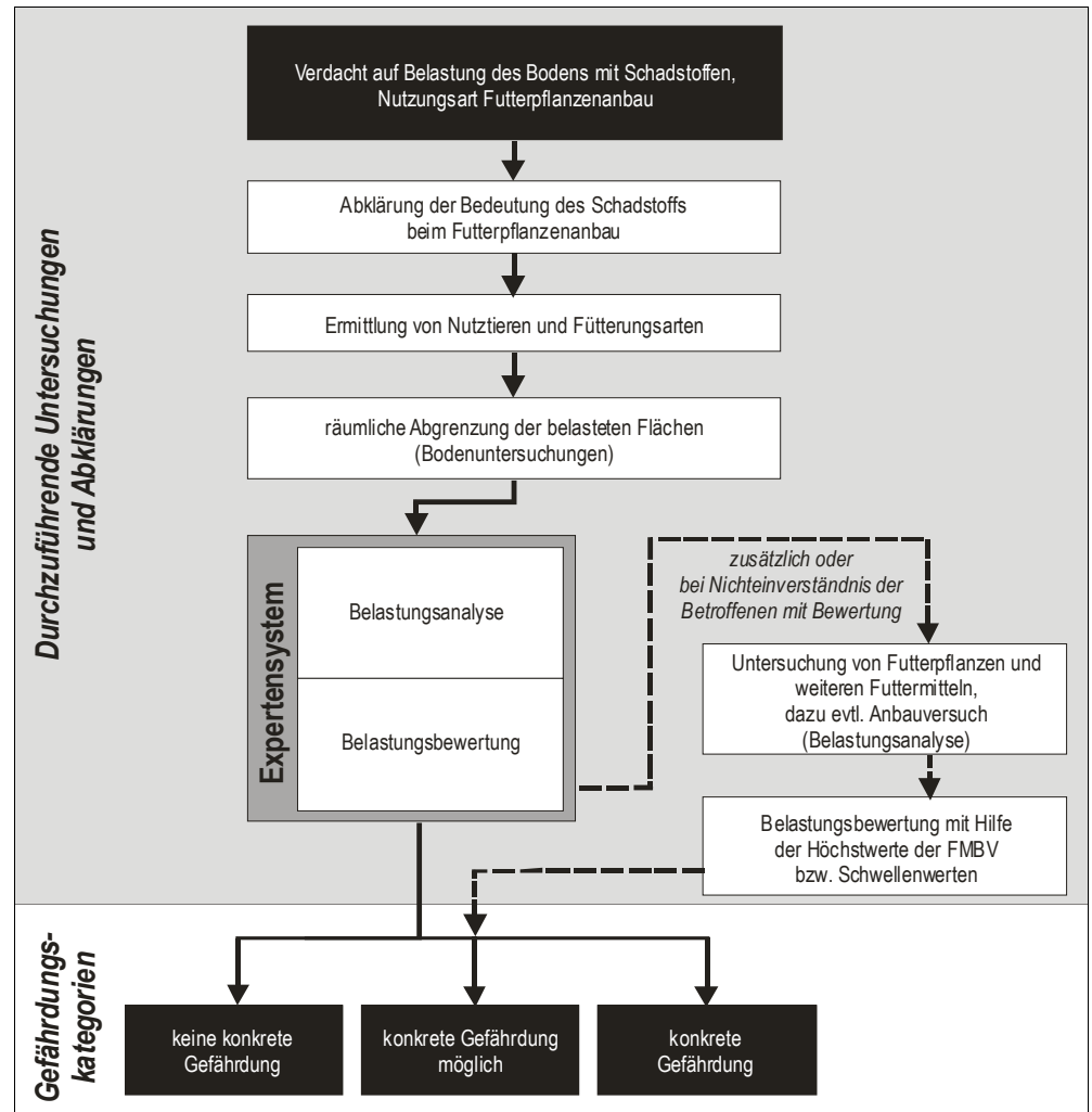
Abb. 5: Das Vorgehen in der Gefährdungsabschätzung beim Futterpflanzenanbau. [FMBV: Futtermittelbuch-Verordnung; SR 916.307.1].
