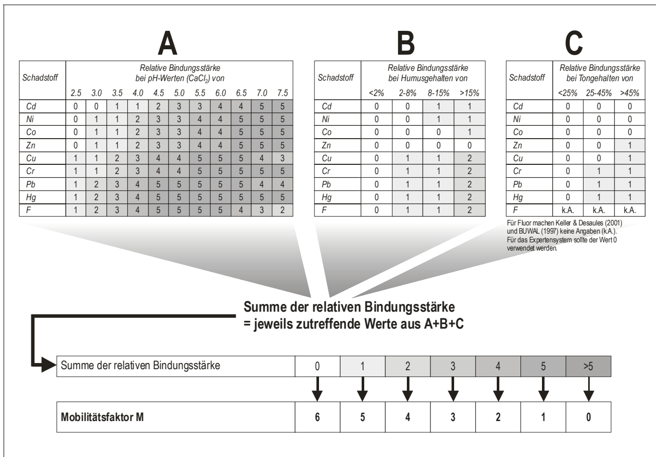
Abb. 4: Ermittlung des Mobilitätsfaktors. Die Werte der Listen A–C wurden aus DVWK (1988) übernommen, ergänzt durch Angaben zu Fluor aus KELLER & DESAULES (2001) und BUWAL (1997c). Laut SCHEFFER & SCHACHTSCHABEL (2002; vgl. S. 369) kann die Mobilität von TI mit jener von Zn und die Mobilität von As mit jener von Cr in etwa verglichen werden.
